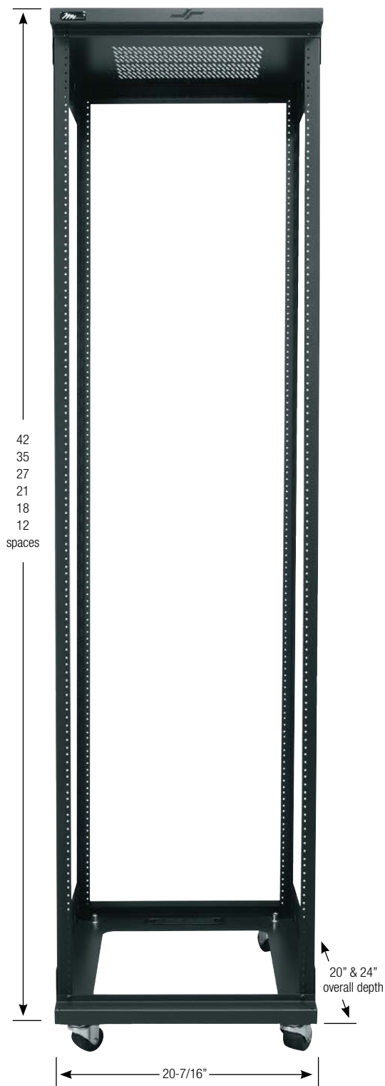
QAR-42-24
