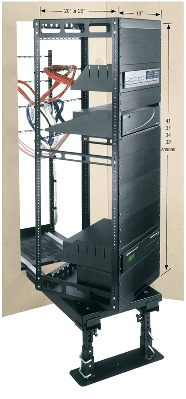
AX-SXR
