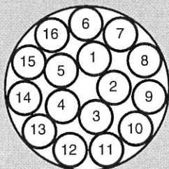
400-PAIR
