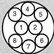
200-PAIR
