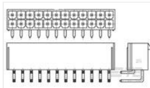
TE Part #2-1586041-2 22P VAL-U-LOK R/A HDR V2
