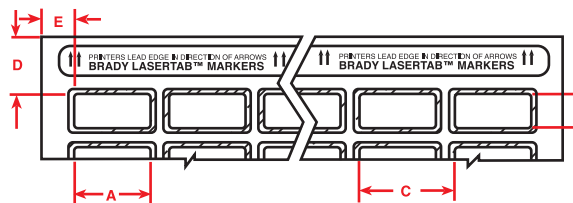
Fig. Laser-05
