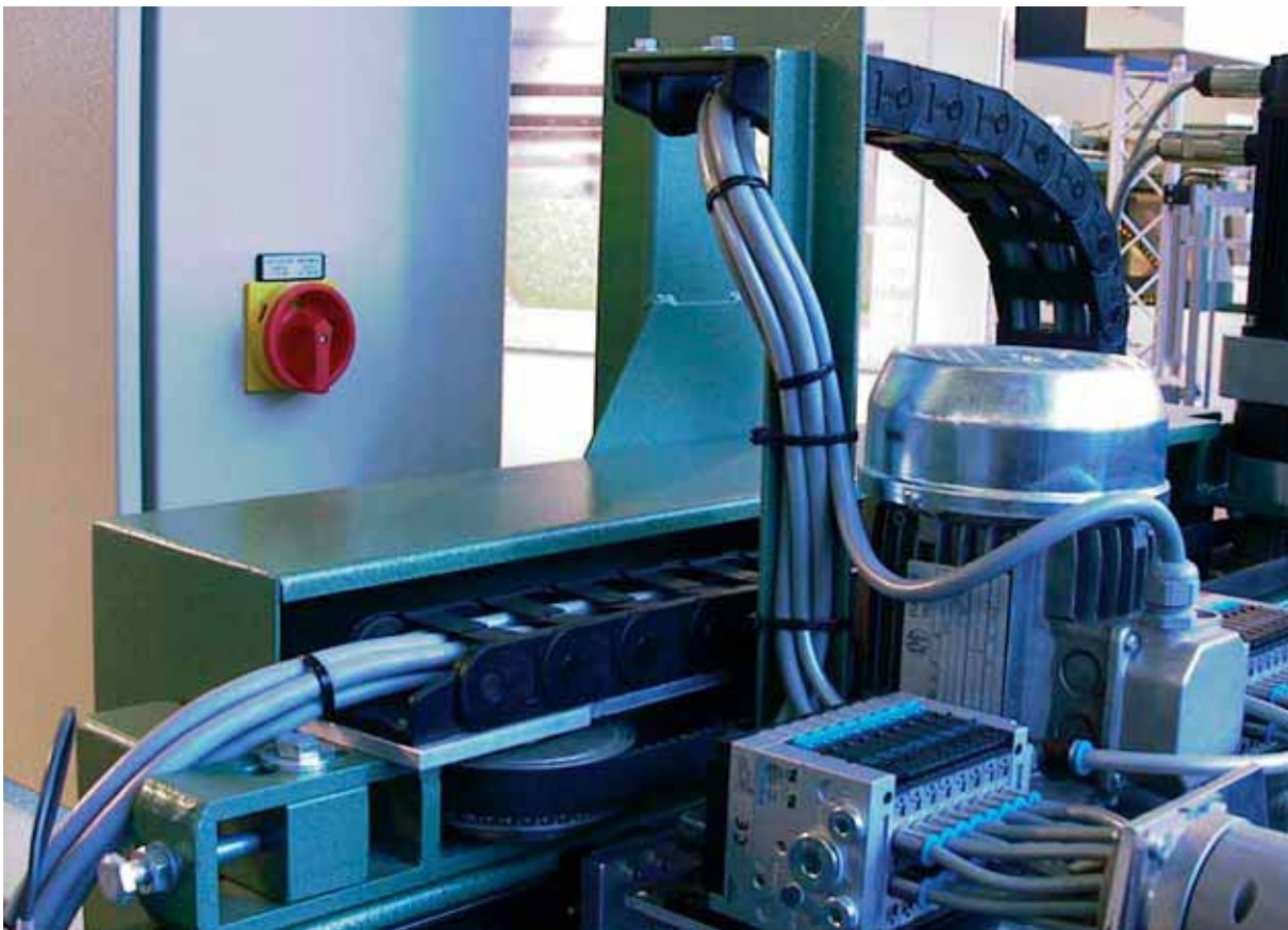
CF140.UL no sistema automático de alimentação. Calha articulada: Easy Chain®
